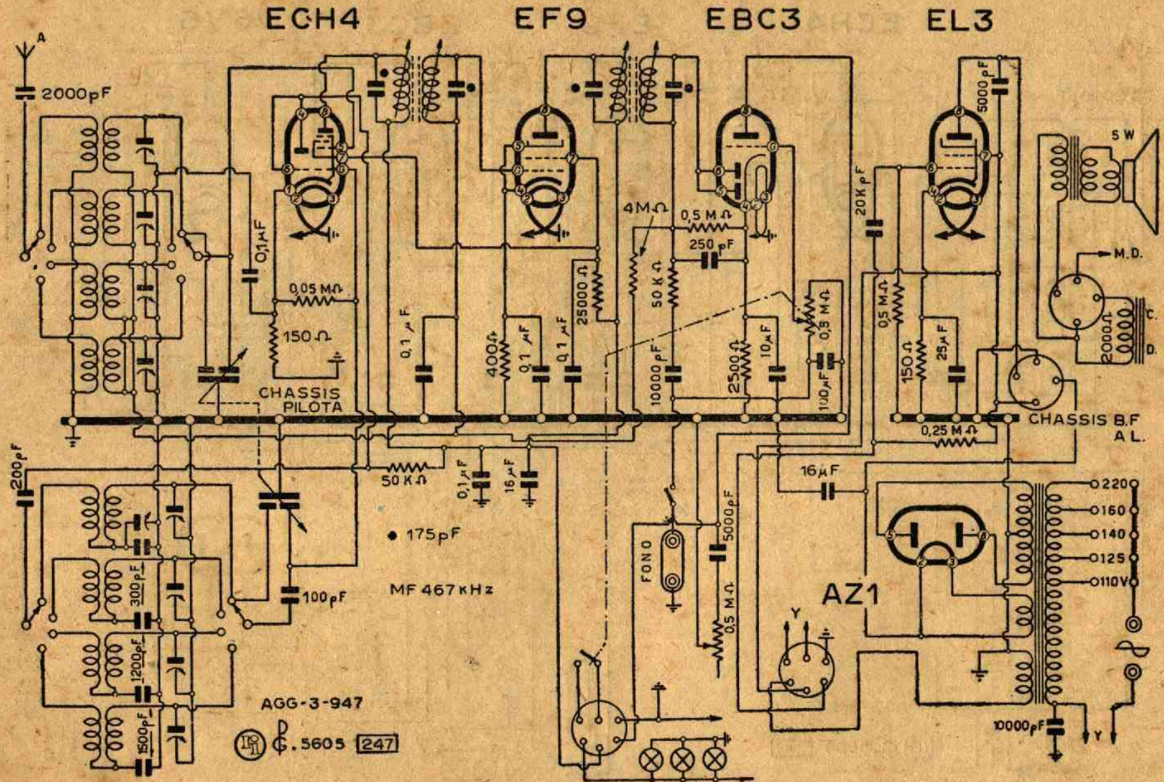
Lo schema elettrico del mod. 542 R
